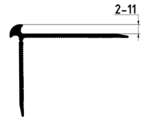
Treppenprofil Stair profile | Profilé d'escalier 8772 - 8779
